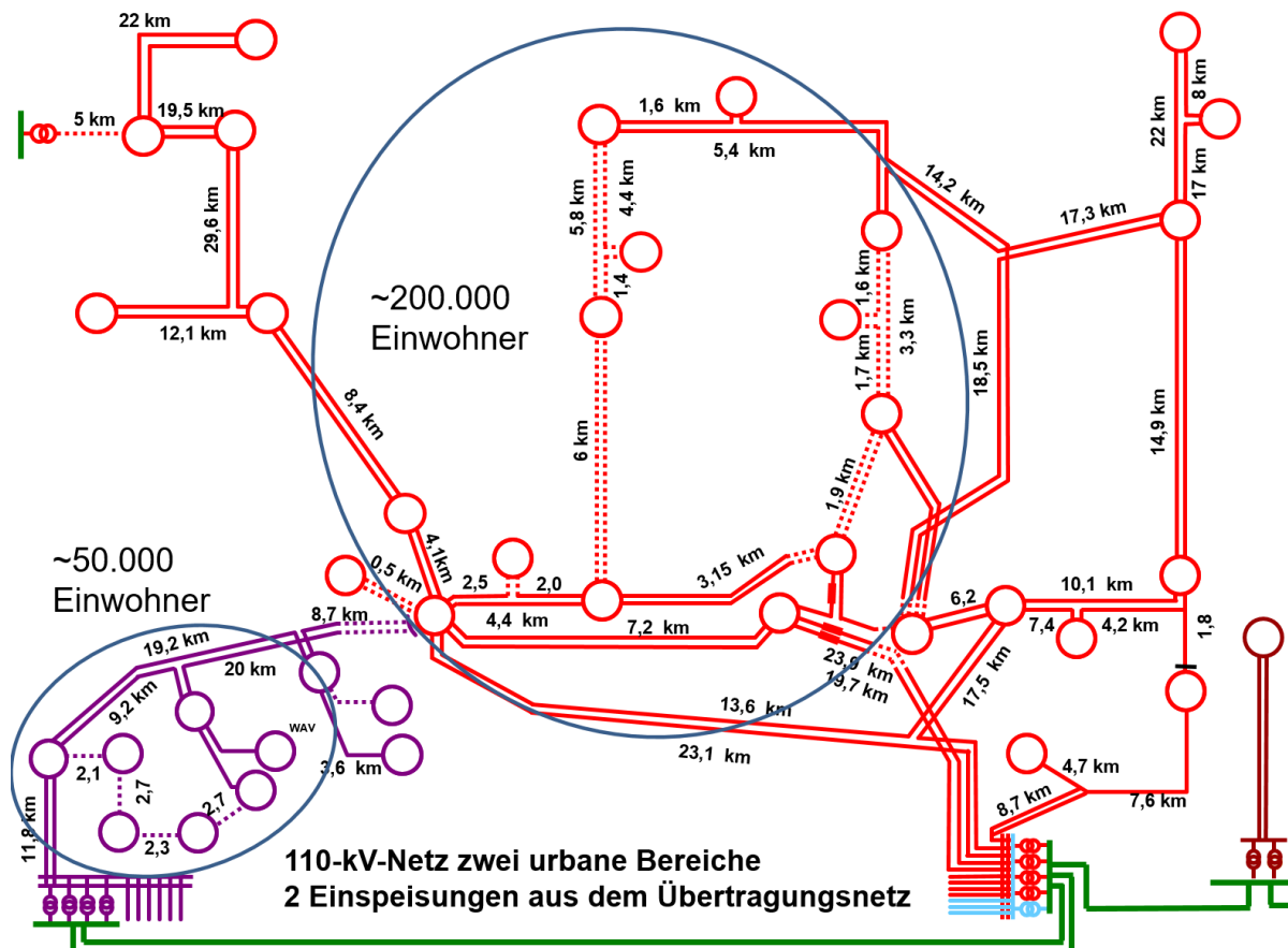
Abbildung: Netztopologie 2018 des östlichen 110-kV-Netzes EAEH in Oberösterreich (Ohne Steyr, Kirchdorf und Traunviertel) mit dem zuschaltbaren Netzabschnitt im Bereich Wels.
