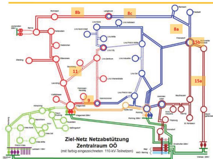
Abbildung: Netztopologie 2026 nach dem Stromnetz-Masterplan OÖ 2026
