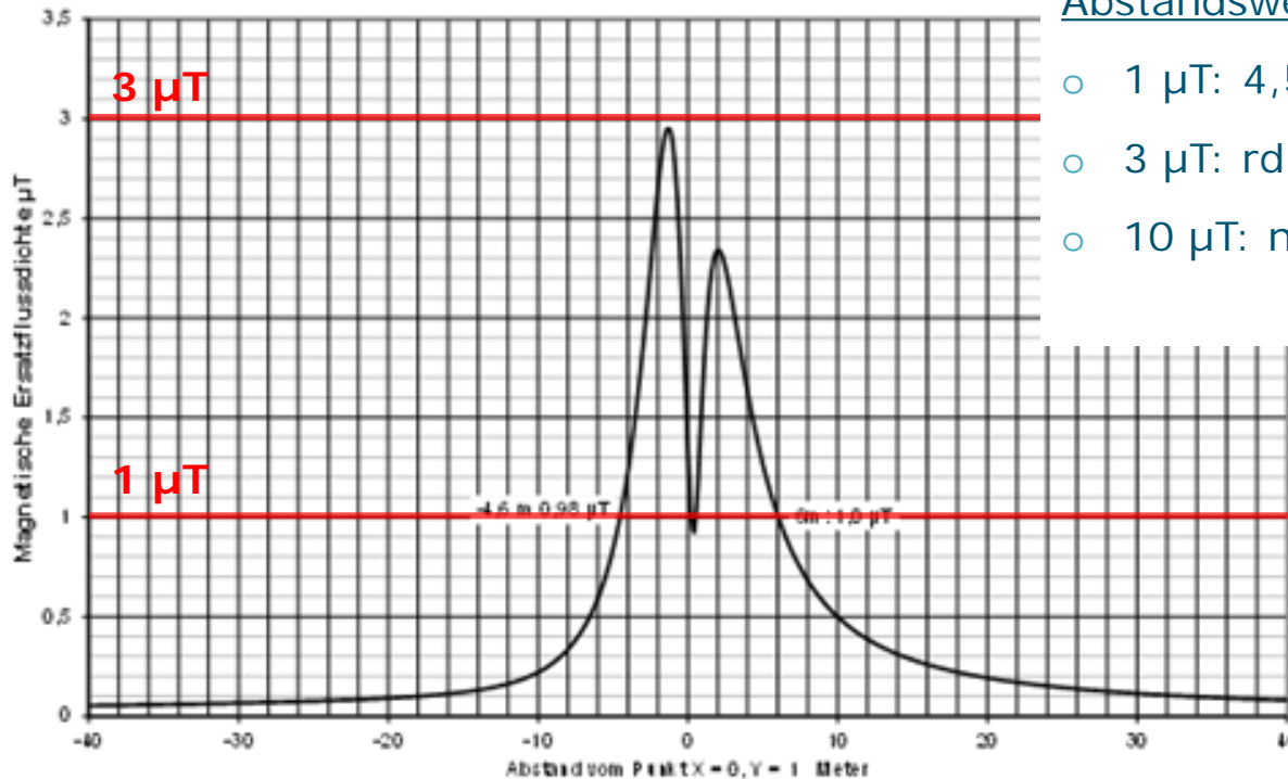
Querprofil magnetische Flussdichte
